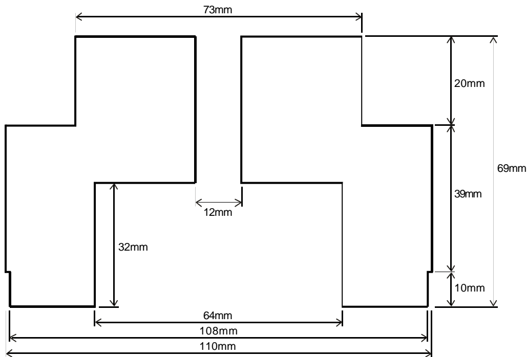
Calço traseiro
